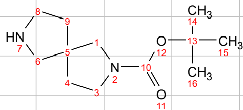
tert-Butyl 2,7-diazaspiro[4.4]nonane-2-carboxylate CAS:236406-49-8
