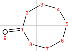
Cyclooctanone CAS:502-49-8
