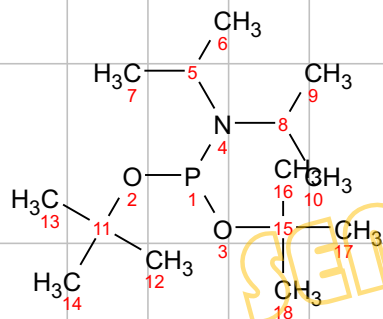
Di-tert-butyl diisopropylphosphoramidite CAS:137348-86-8
